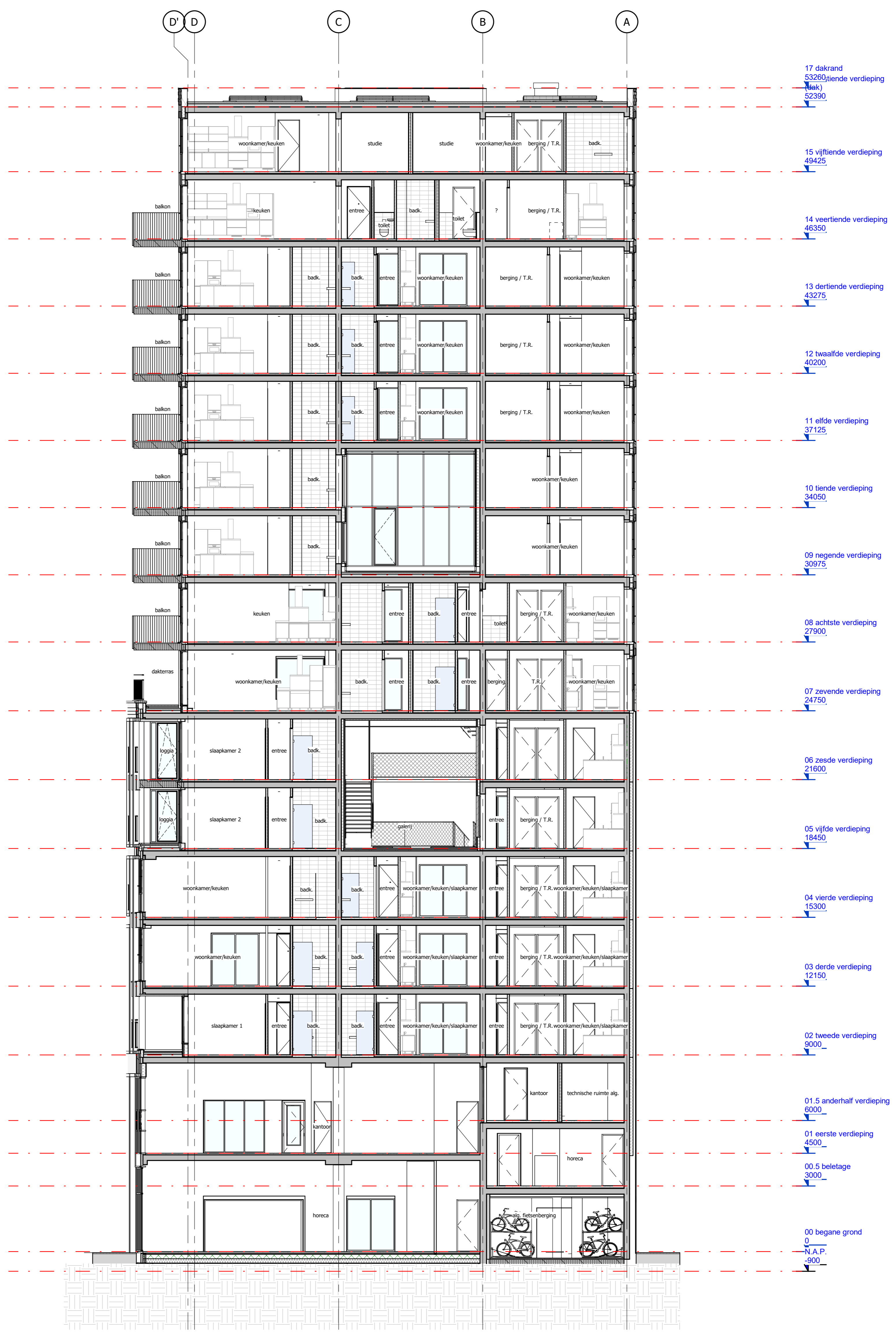
Doorsnede D1
