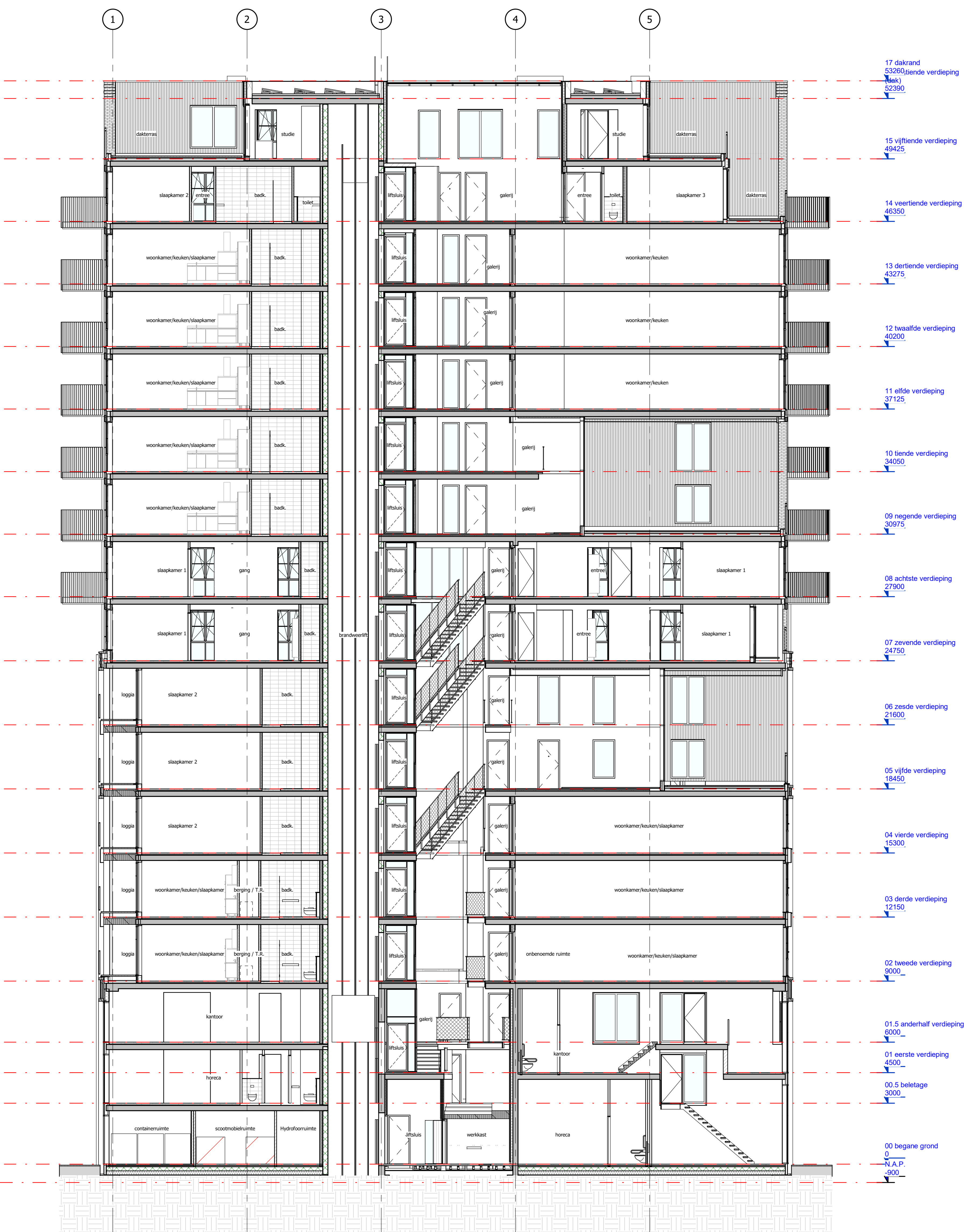
Doorsnede B
