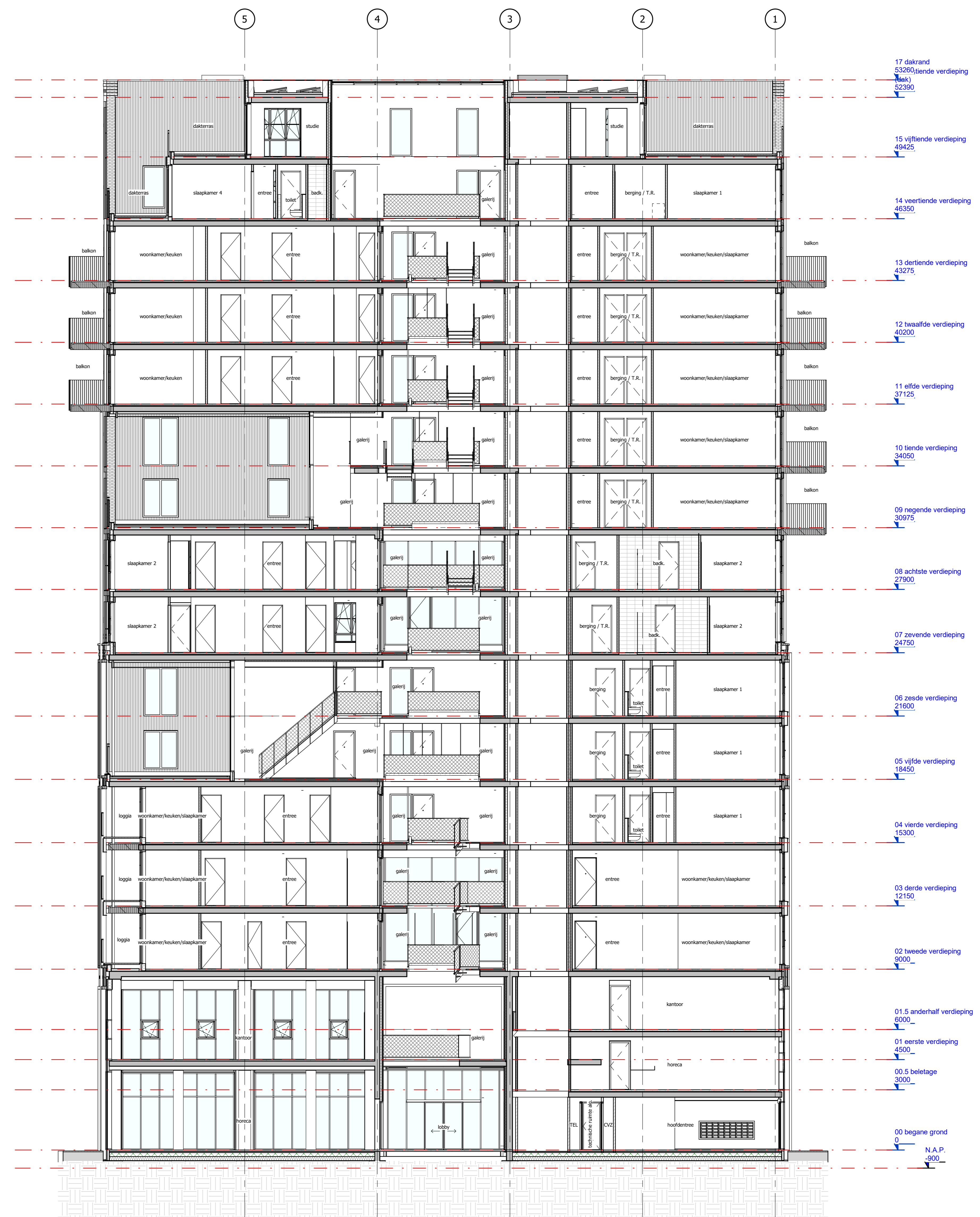
Doorsnede B1
