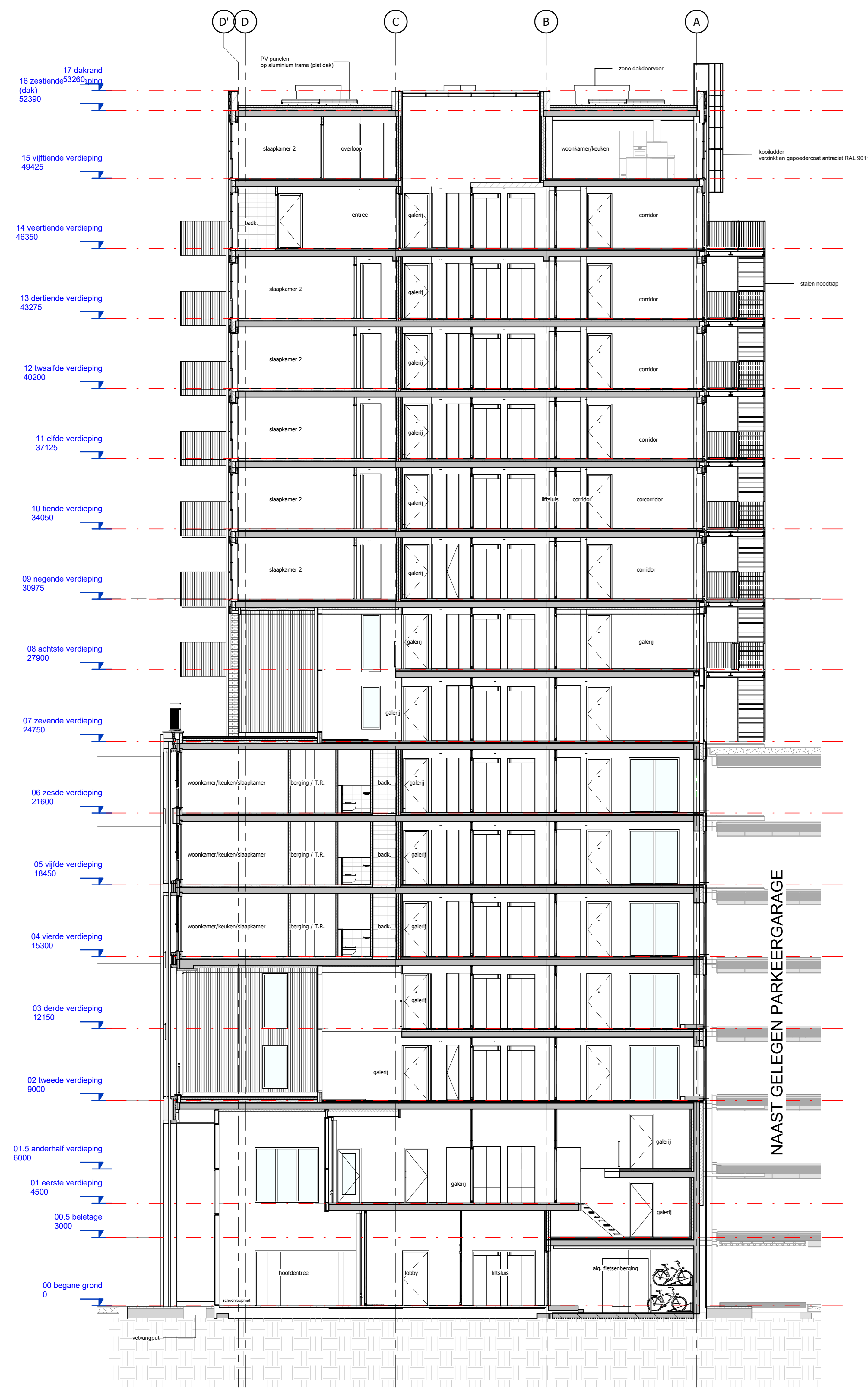
Doorsnede A
