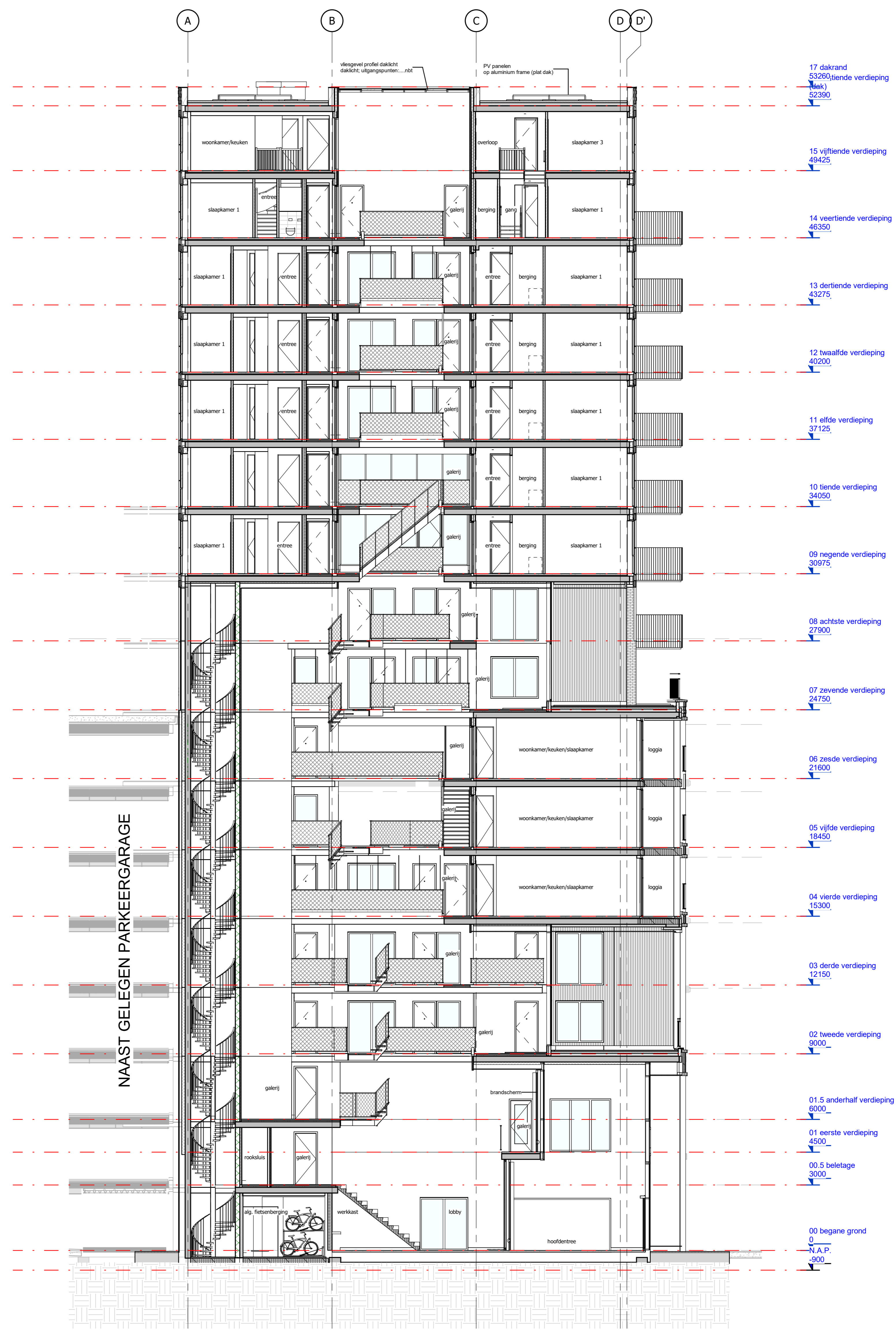
Doorsnede A1
