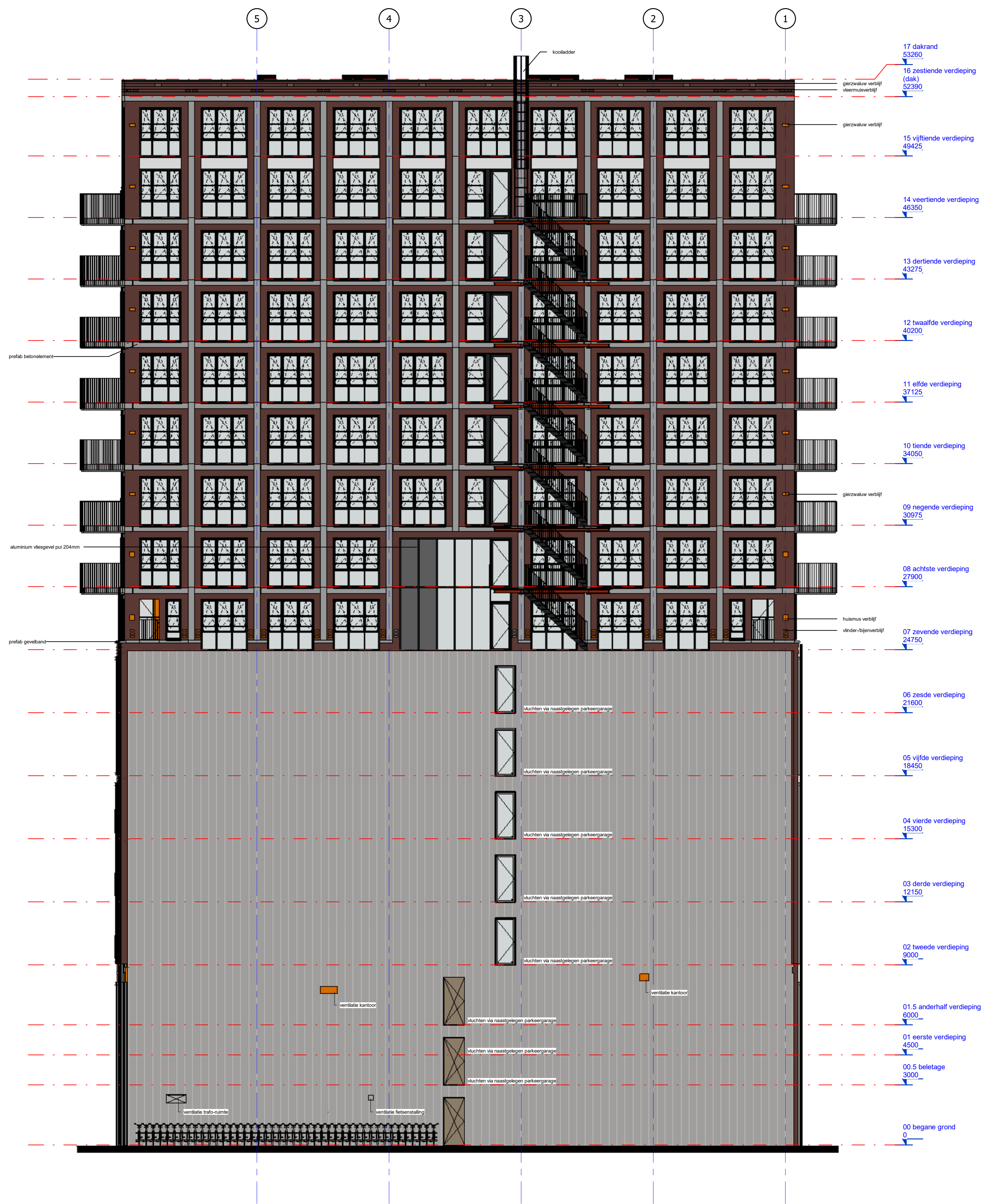
NO-gevel (as-A)
