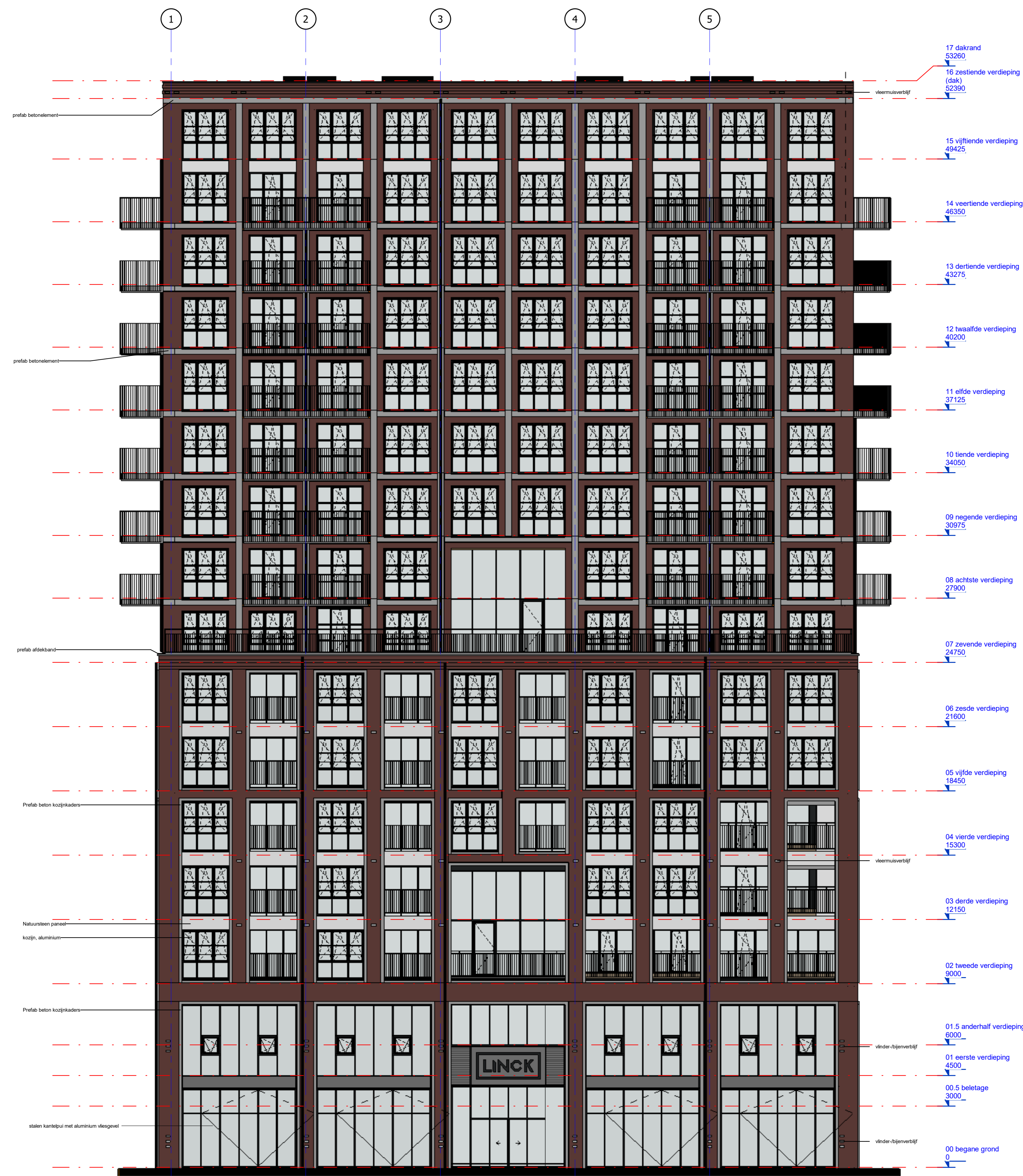
ZW-Gevel (as-E)
