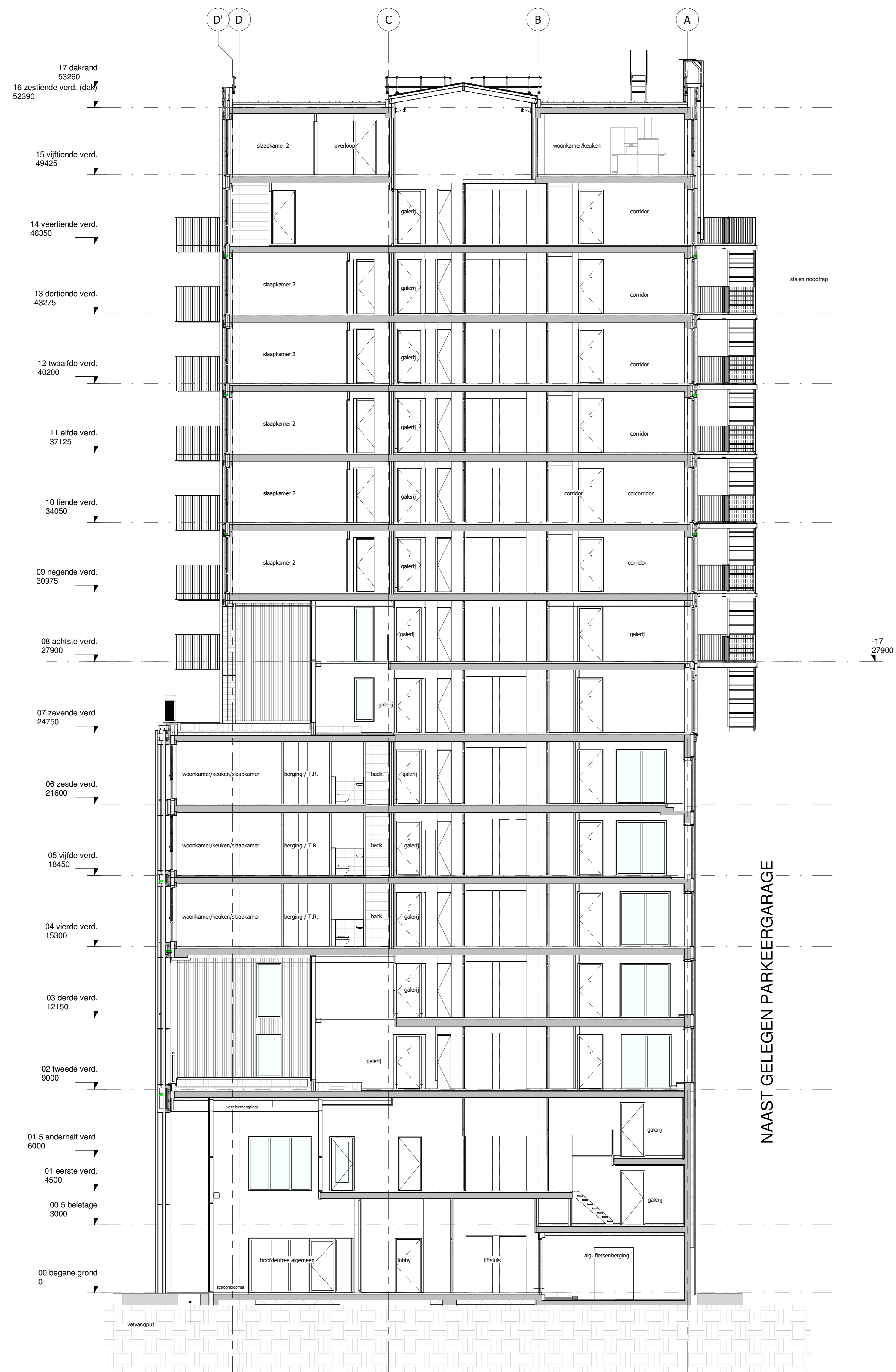
Doorsnede A
