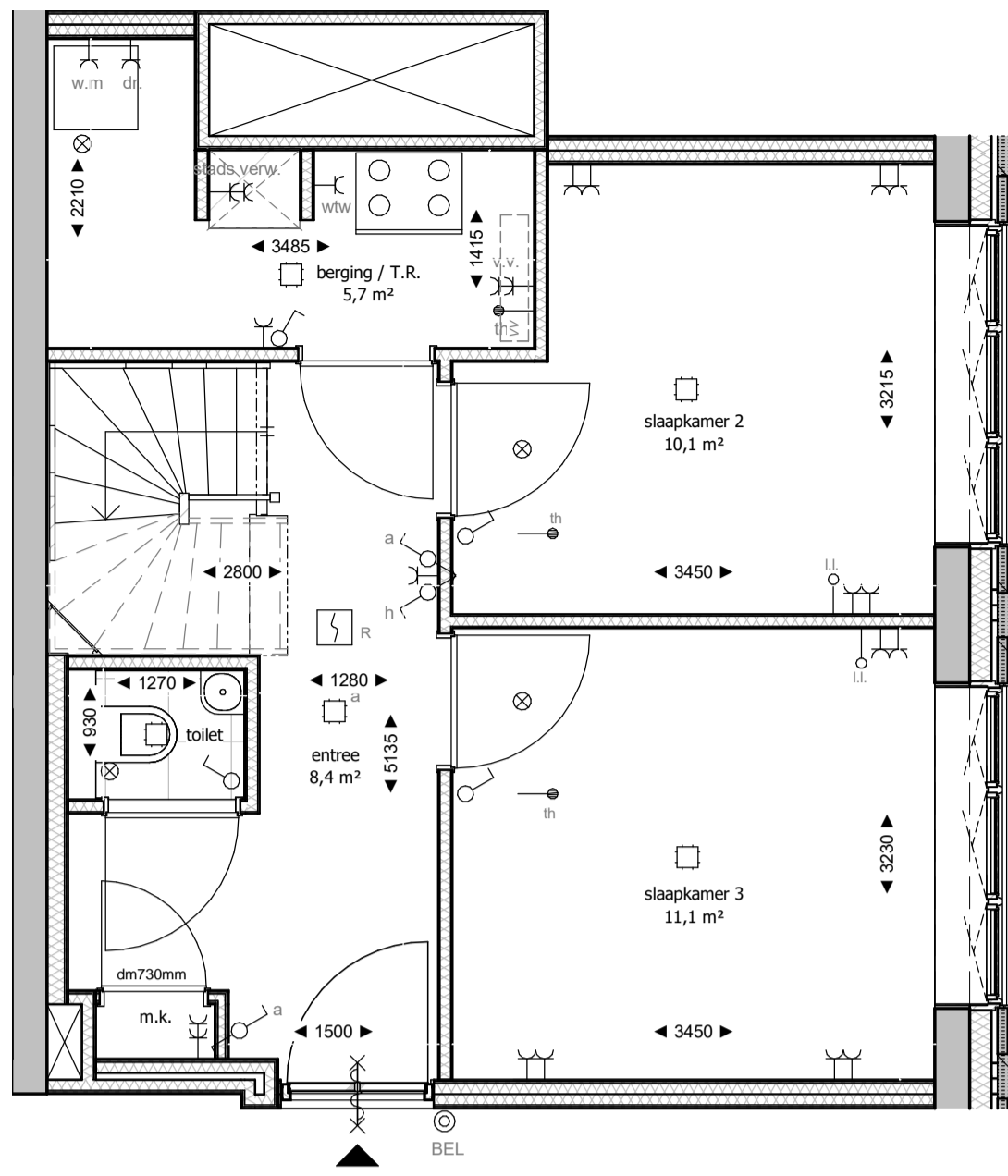
Veertiende verdieping
